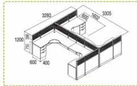
TY-WS024 ชุด Workstation 4 ที่นั่ง 3305(W) x 3280(D) x 1200(H) mm.
