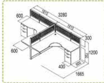
TY-WS012 ชุด Workstation 2 ที่นั่ง 3280(W) x 1665(D) x 1200(H) mm.
