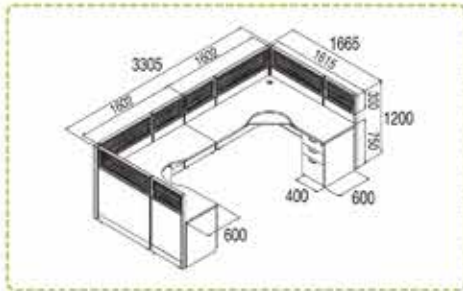
TY-WS022 ชุด Workstation 2 ที่นั่ง 3305(W) x 1665(D) x 1200(H) mm.
