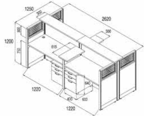
TY-WS044 ชุด Workstation 4 ที่นั่ง 2620(W) x 1250(D) x 1200(H) mm.
